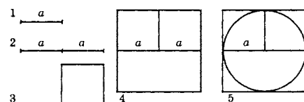
Рис. 1.3. Алгоритм построения окружности с заданным радиусом
